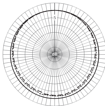
— 1 kHz - - - - 10 kHz - - - - 12.5 kHz
