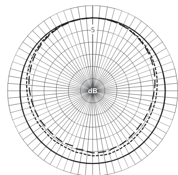
— 1 kHz - - - - 16 kHz - - - - 20 kHz
